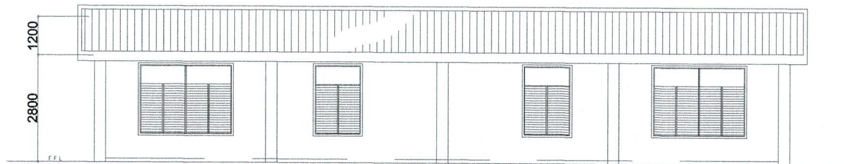
REAR ELEVATION SCALE: 1/250
