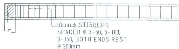
ROOF BEAM DET.
