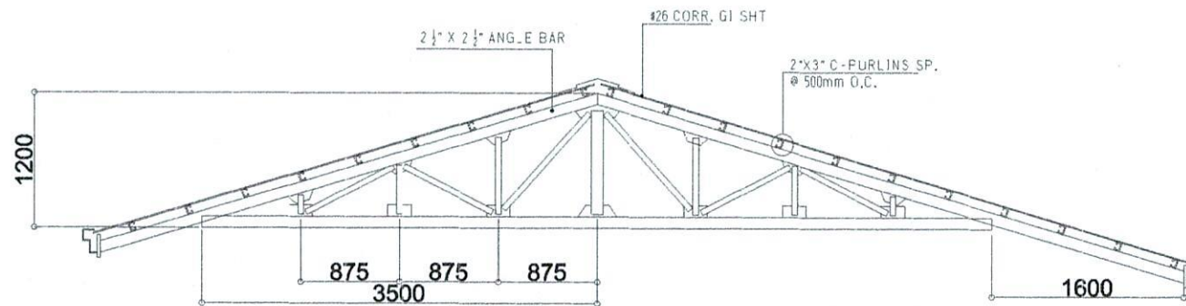
TRUSS DET. SCALE: 3/8"=1'-0"
