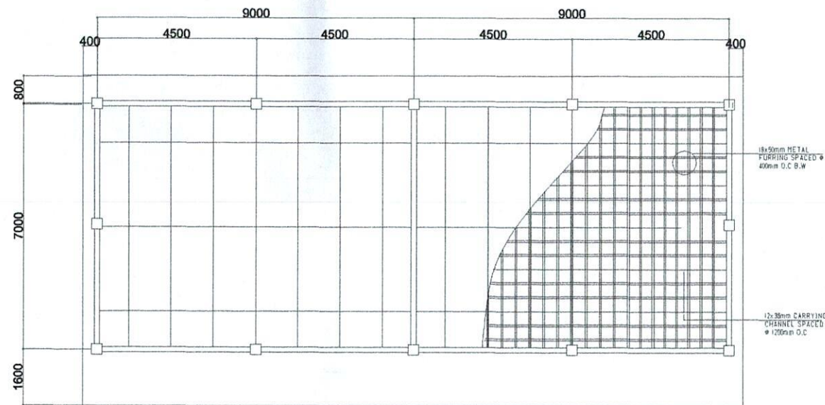
CEILING PLAN SCALE: 1/200
