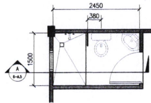
5 SEMI-PRIV. TOILET PLAN SCALE 1:16 M
