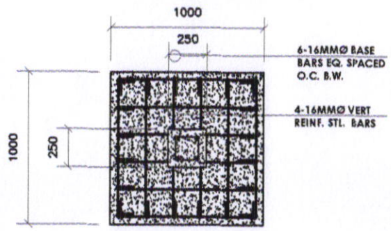
C1F1 PLAN & SECTION AD-00 SCALE N.T.S.
