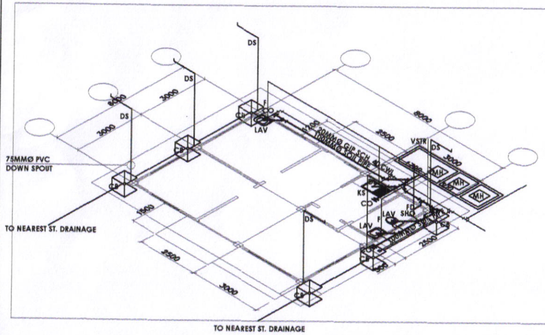
ISOMETRIC LAYOUT AD-00 SCALE N.T.S.
