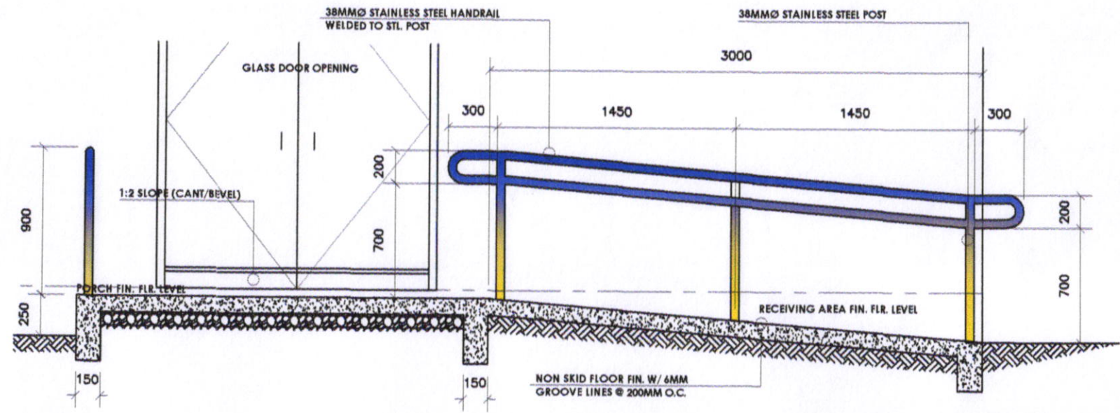
DET. SECTION OF RAMP & PORCH AD-00 SCALE N.T.S.
