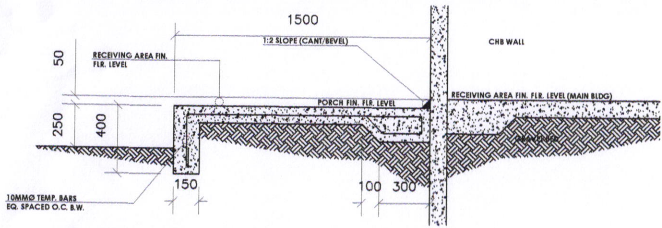
DET. SECTION OF PORCH AD-00 SCALE N.T.S.
