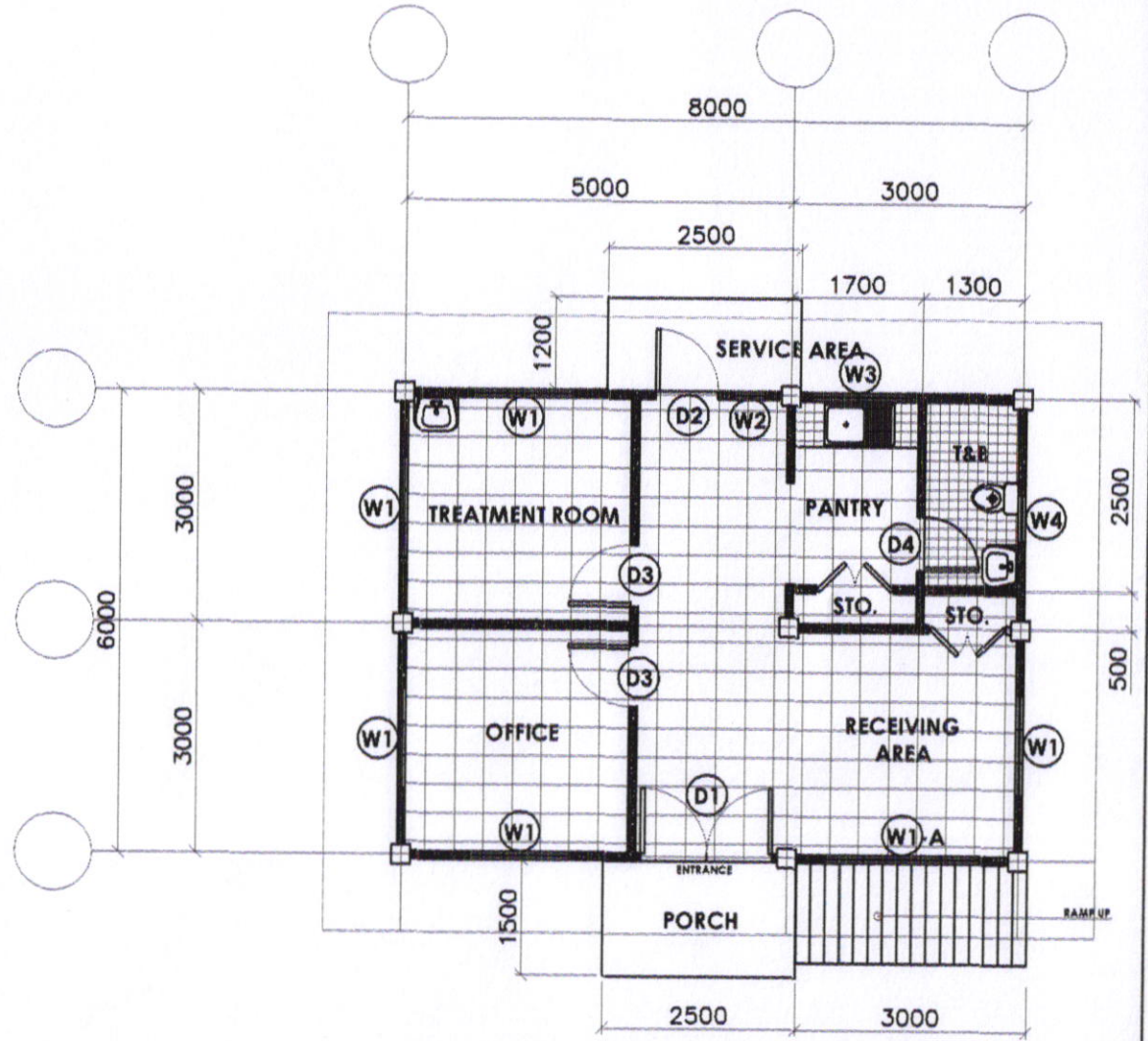
FLOOR PLAN AD-00 SCALE N.T.S.
