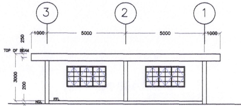
LEFT SIDE ELEVATION SCALE: 1:100MTS
