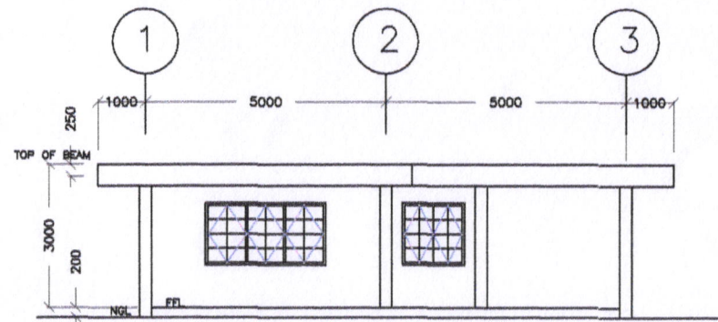
RIGHT SIDE ELEVATION SCALE: 1:100MTS
