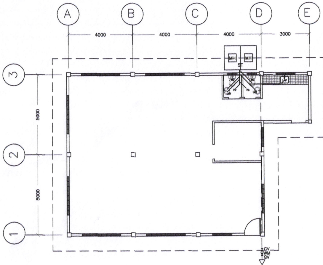
PLUMBING LAYOUT SCALE: 1:100MTS
