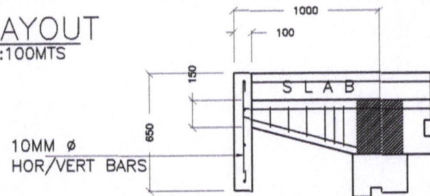
LENTEL BEAM DET. SCALE: 1:30MTS
