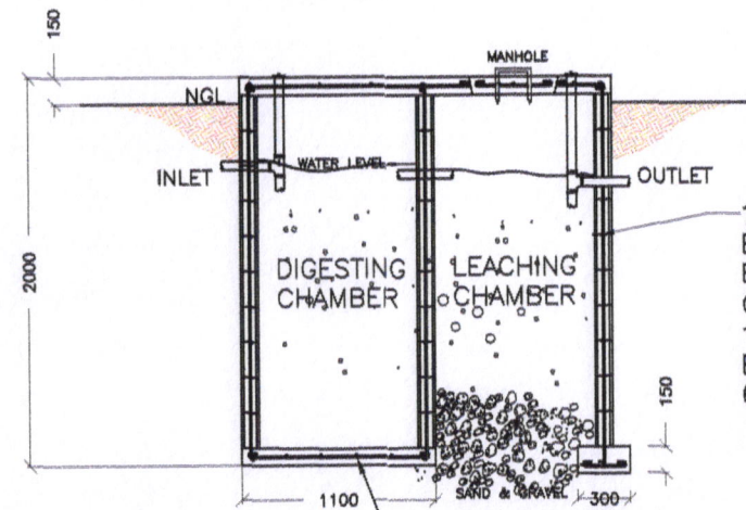
SEPTIC TANK DET. SCALE: 1:50MTS
