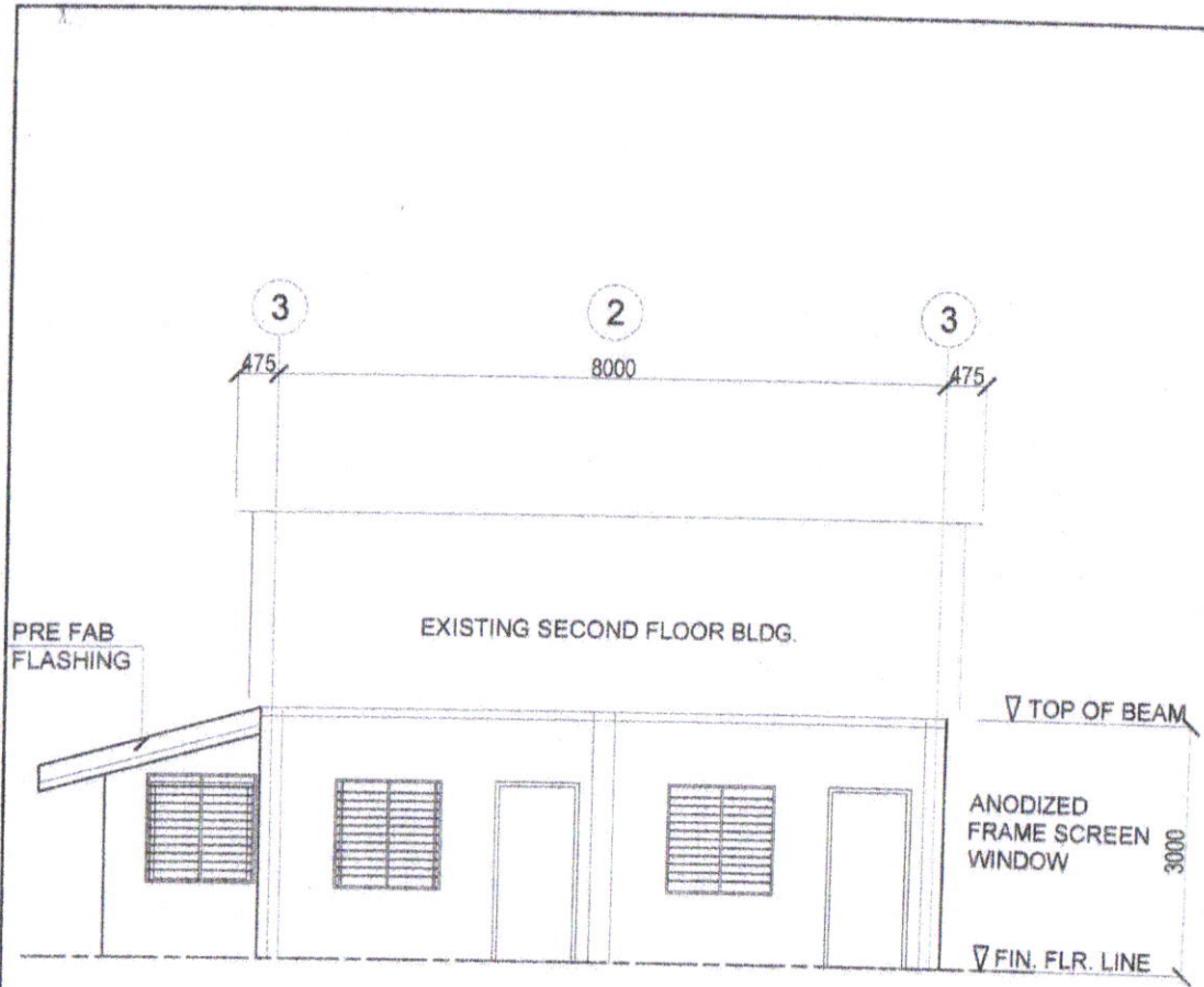
FRONT ELEVATION SCALE: 1:100M.
