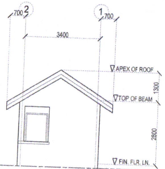
FRONT ELEVATION SCALE: 1:100M.
