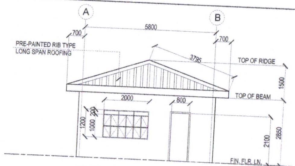
FRONT ELEVATION SCALE: 1:100M.
