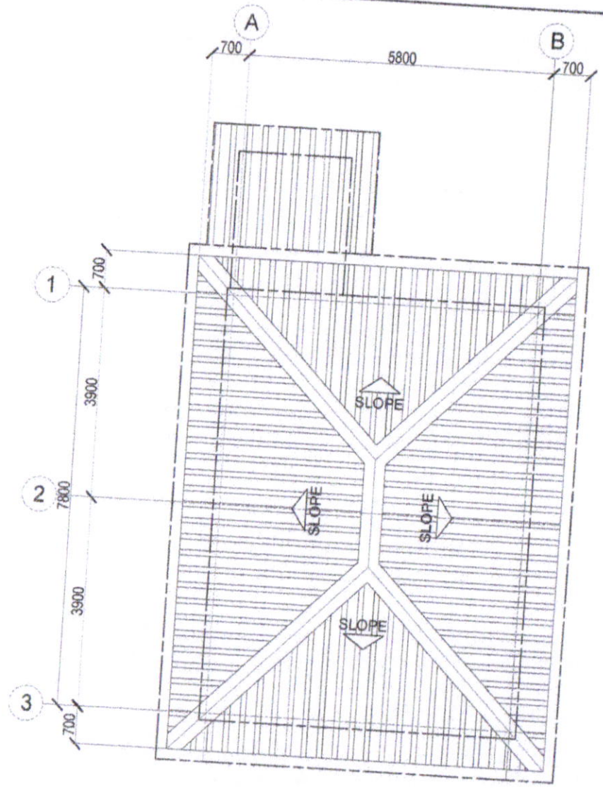
ROOF PLAN SCALE: 1:100M.
