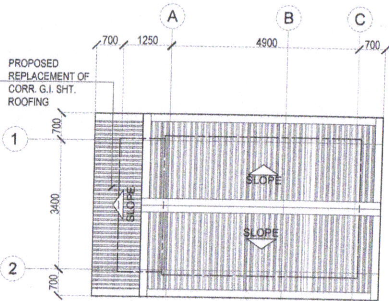
ROOF PLAN SCALE: 1:100M.
