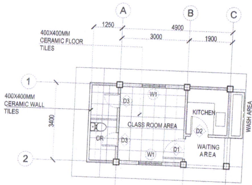
FLOOR PLAN SCALE: 1:100M.
