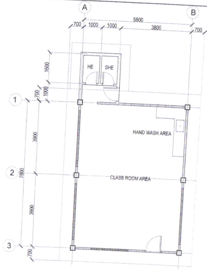
FLOOR PLAN SCALE: 1:100M.
