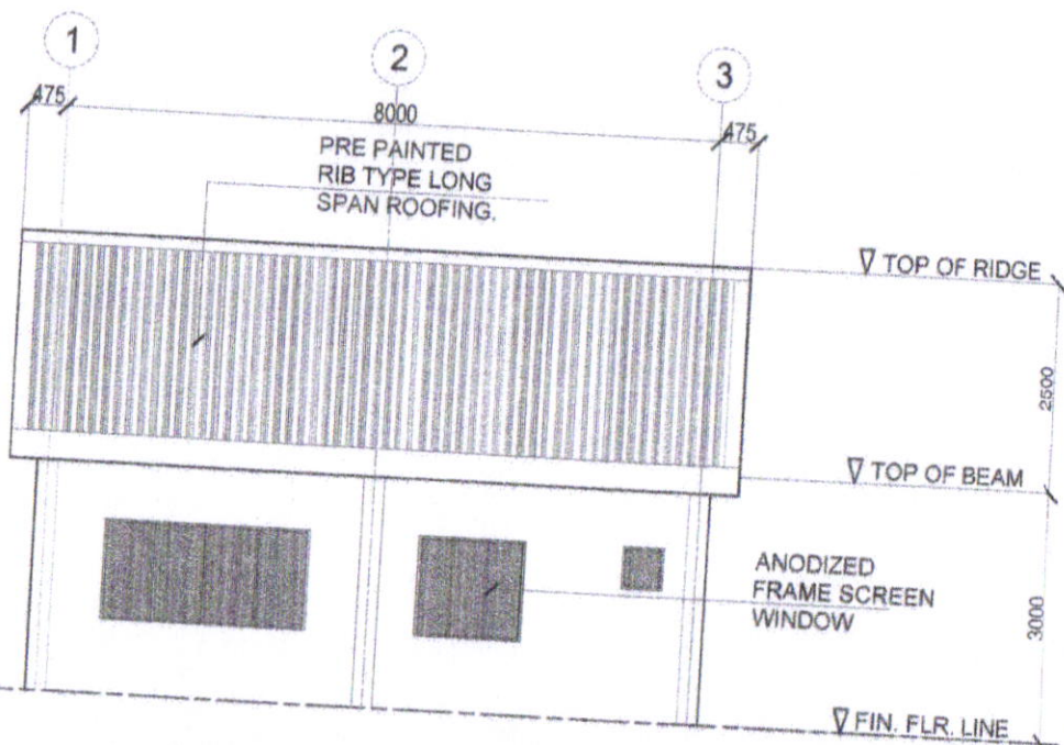
REAR ELEVATION SCALE: 1:100M.
