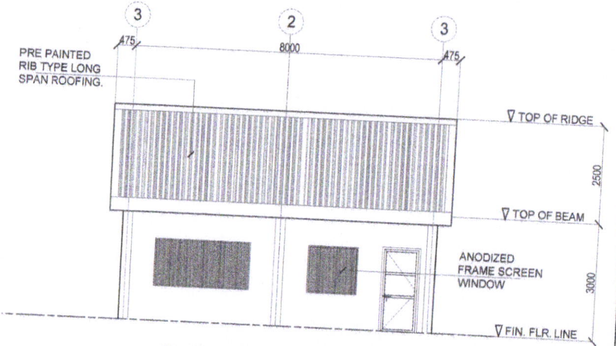
FRONT ELEVATION SCALE: 1:100M.
