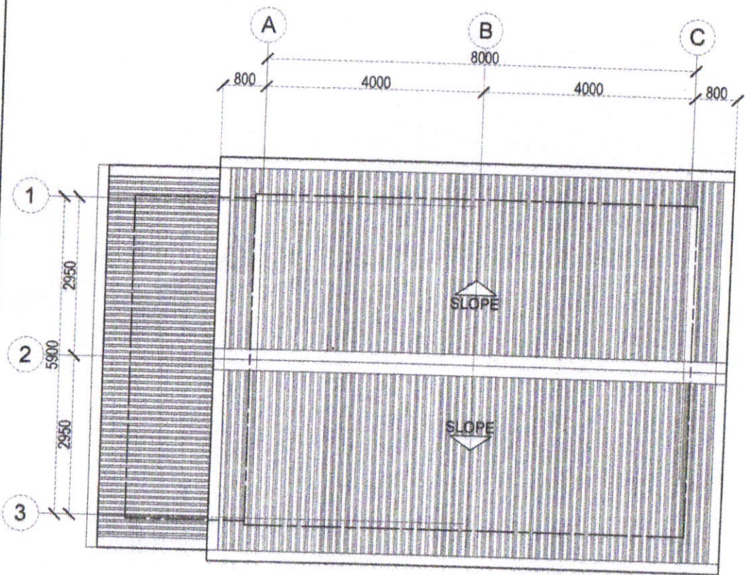
ROOF PLAN SCALE: 1:100M.
