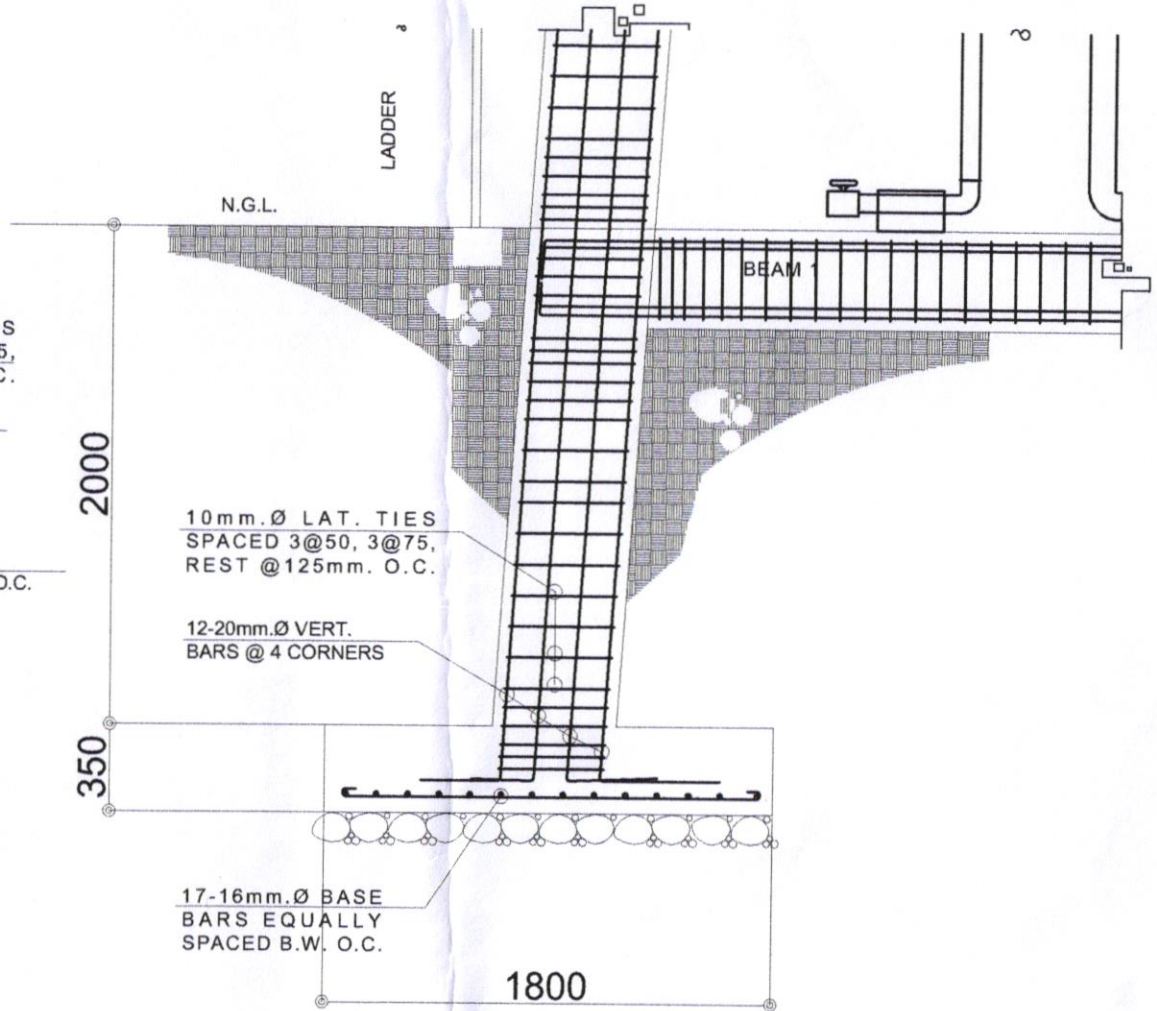
CF SECTION 1:30m.
