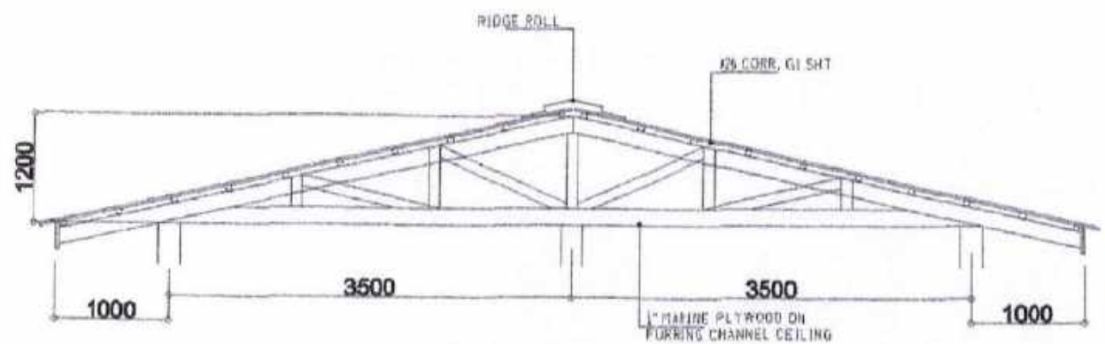
TRUSS DET. SCALE: 1:25RTS
