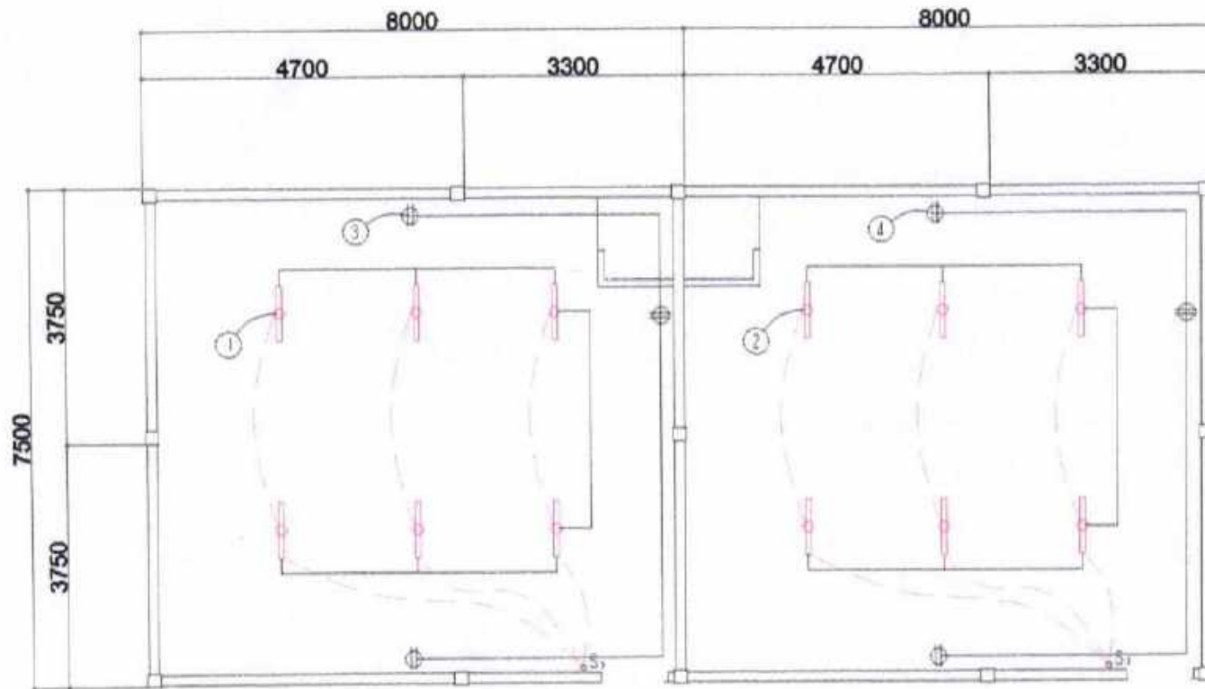
ELECTRICAL PLAN SCALE: 1/8" = 1'-0"
