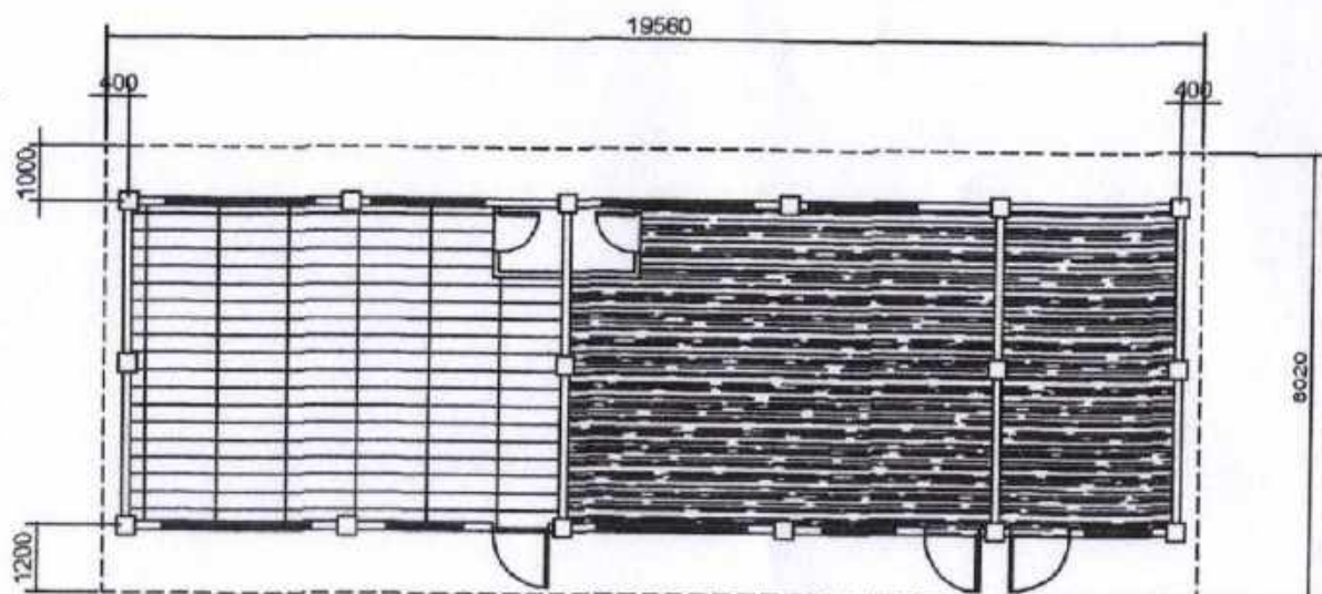
R O O F F R A M I N G P L A N SCALE: N T S
