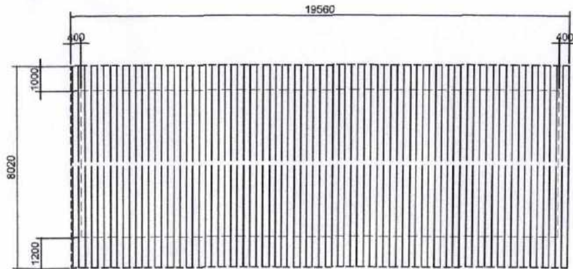
R O O F P L A N SCALE: N T S
