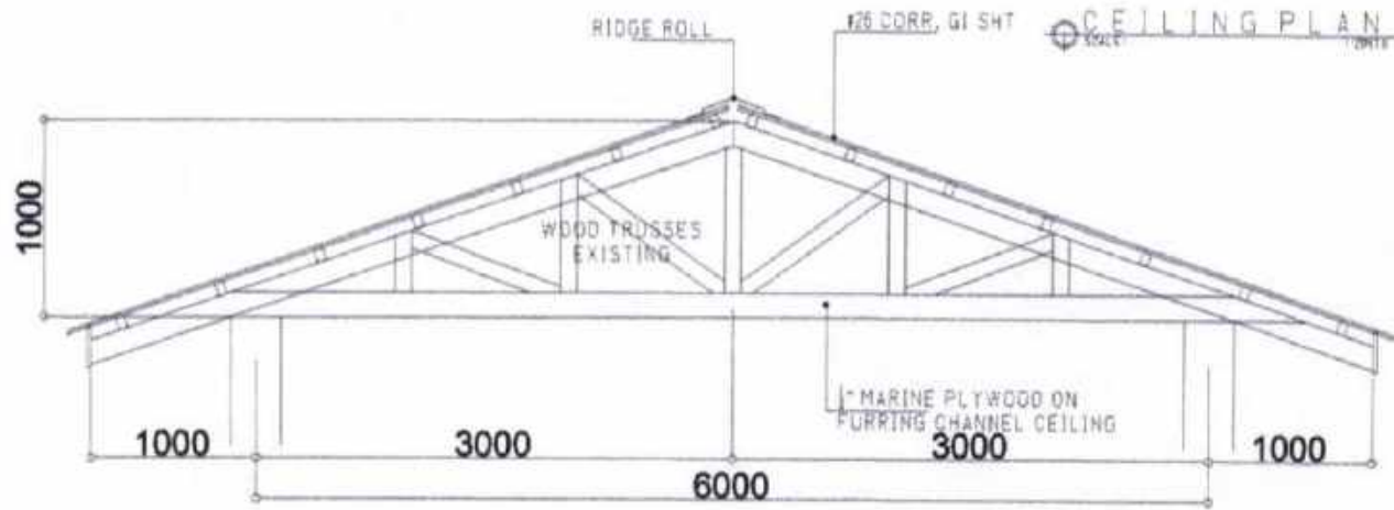
TRUSS DET. SCALE: 1:25PTS
