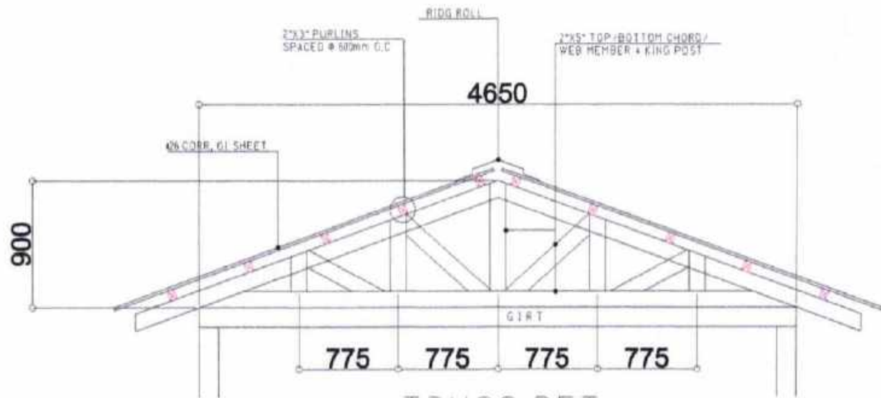
TRUSS DET. SCALE: 1:25MTS
