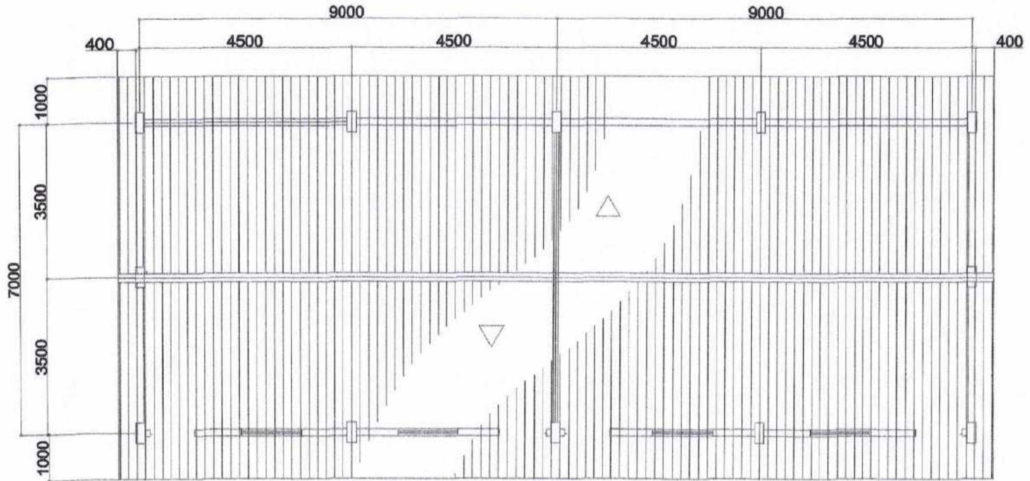
R O O F P L A N
