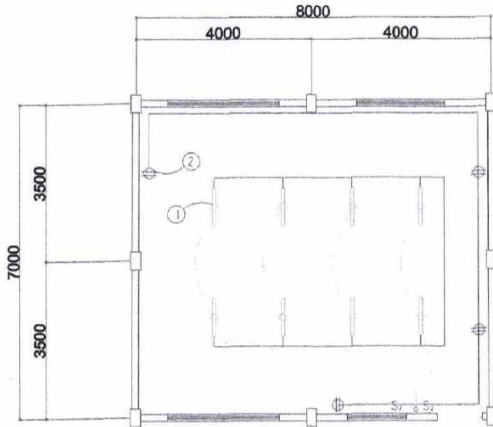
ELECTRICAL PLAN SCALE: 1:200
