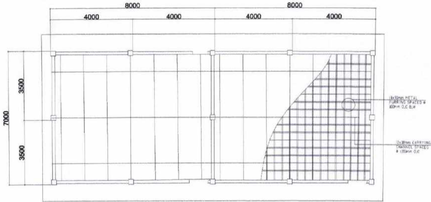
CEILING PLAN SCALE: 1:25 H.T.S.
