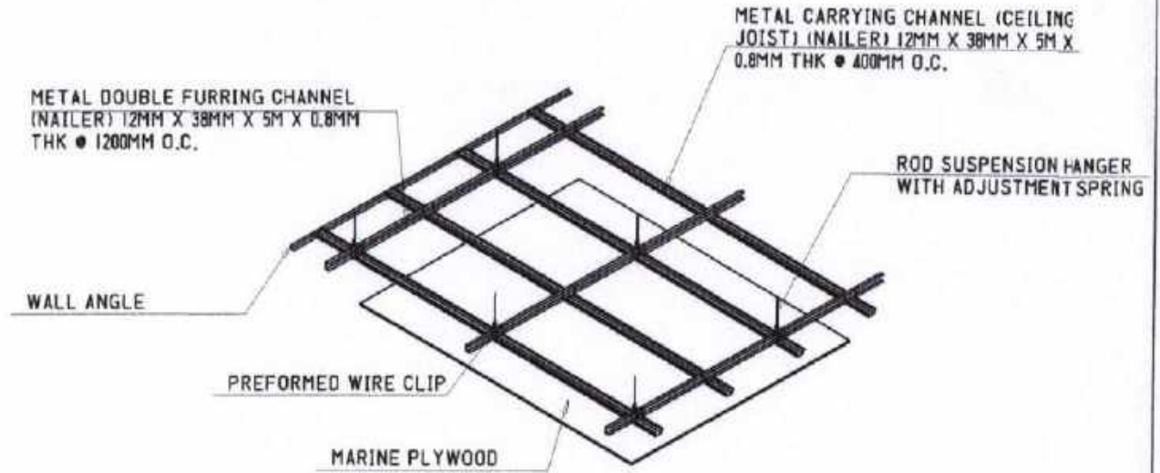
○ CEILING DET. SCALE: N T S
