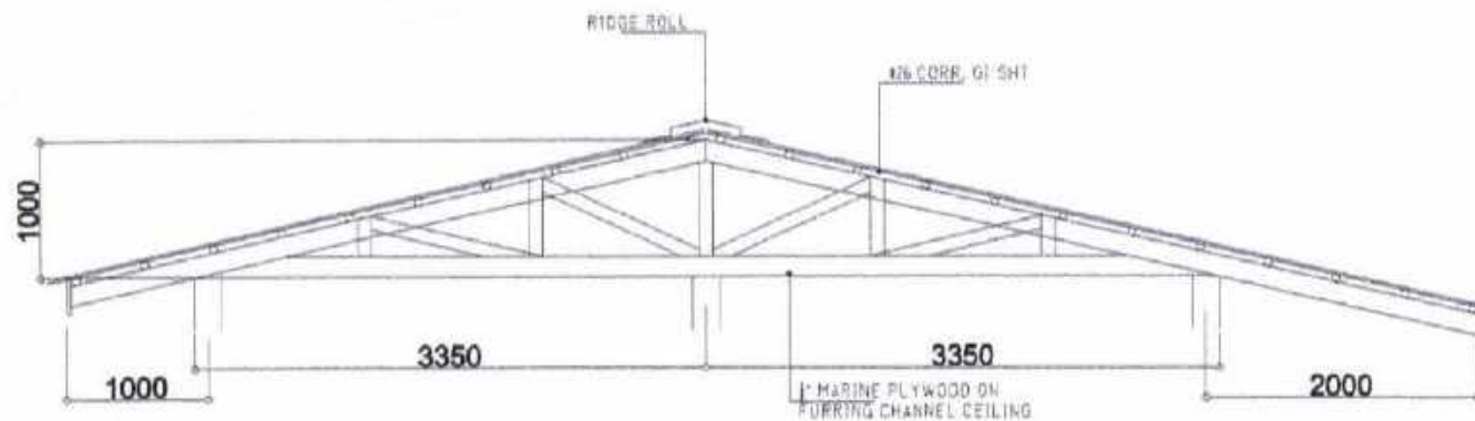
TRUSS DET. SCALE: 1:25M.T.S
