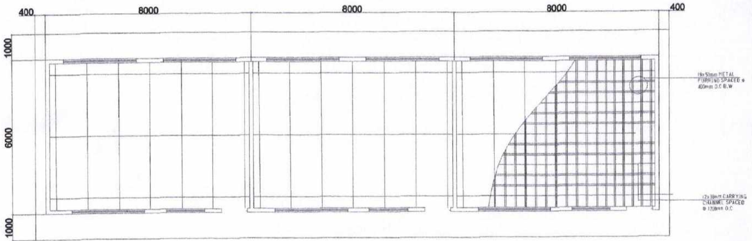
CEILING PLAN SCALE: 1/8"=1'-0"
