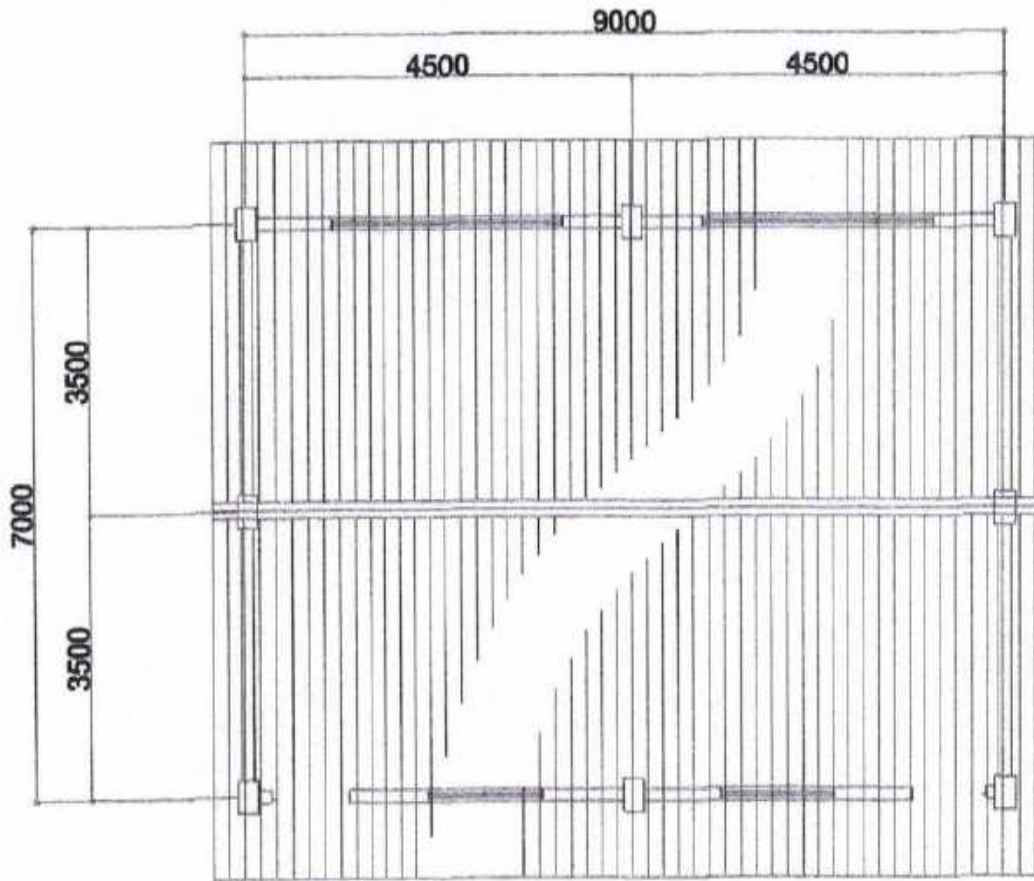
ROOF PLAN SCALE: 1:200
