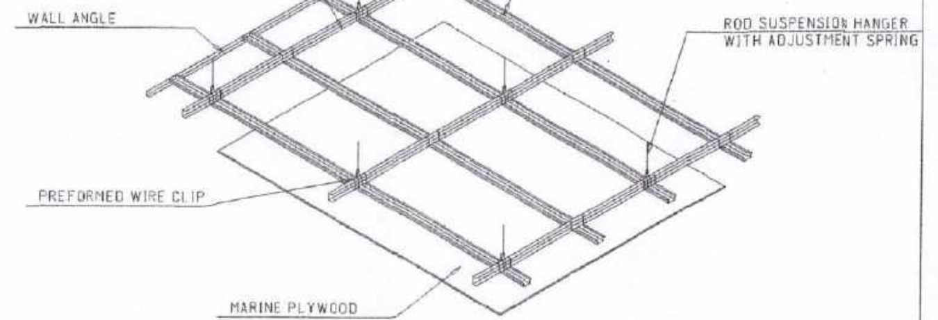
CEILING DET. SCALE: N T S
