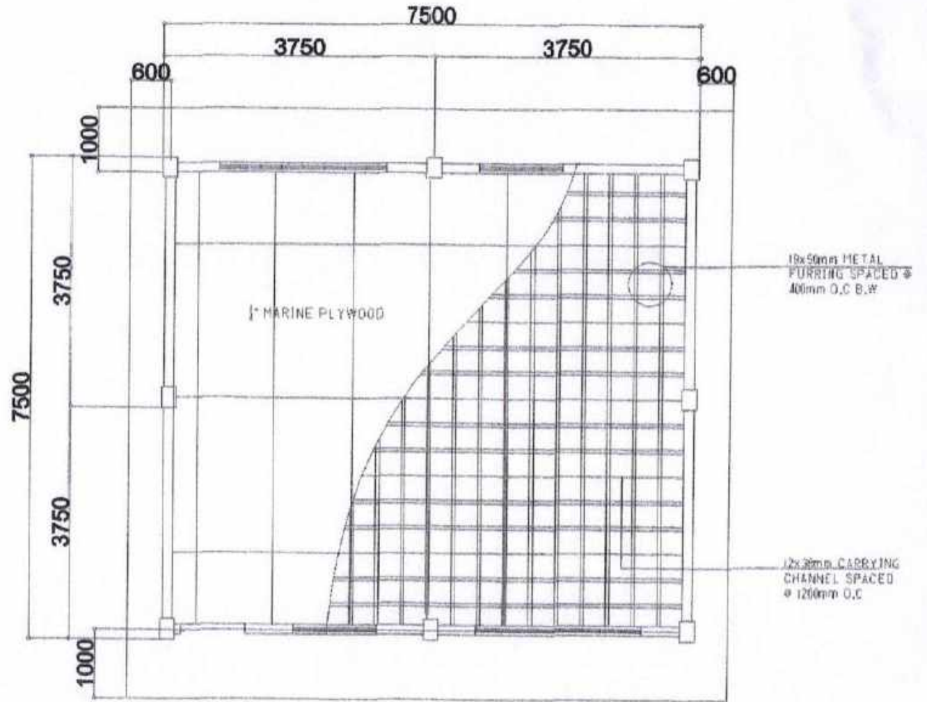
CEILING PLAN SCALE: 1/8"=1'-0"
