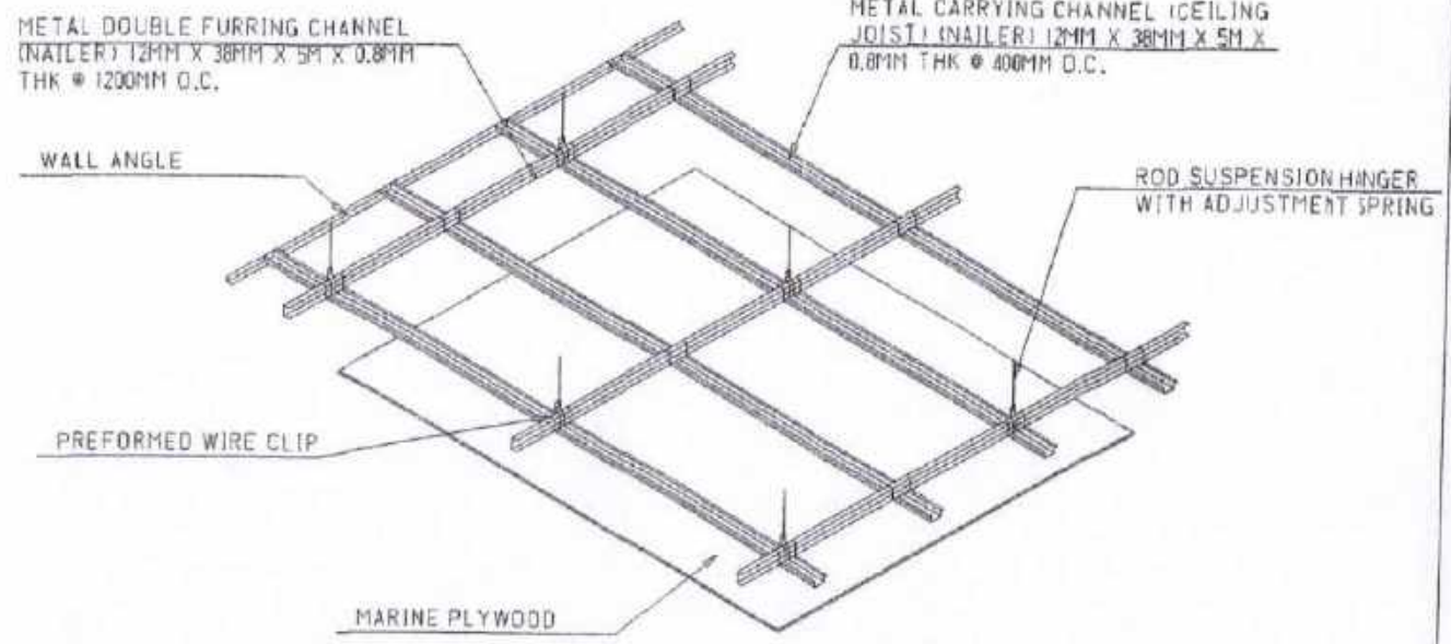
C E I L I N G D E T . SCALE: N T S
