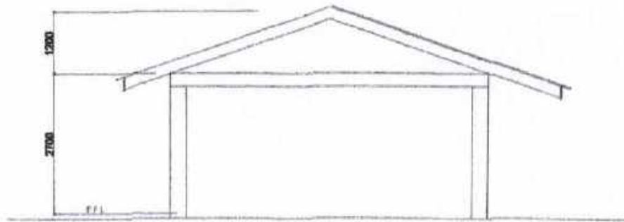
RIGHT SIDE ELEV. SCALE: 1:25MTS
