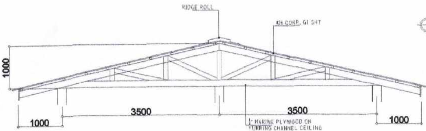
TRUSS DET. SCALE: 1:25HTS
