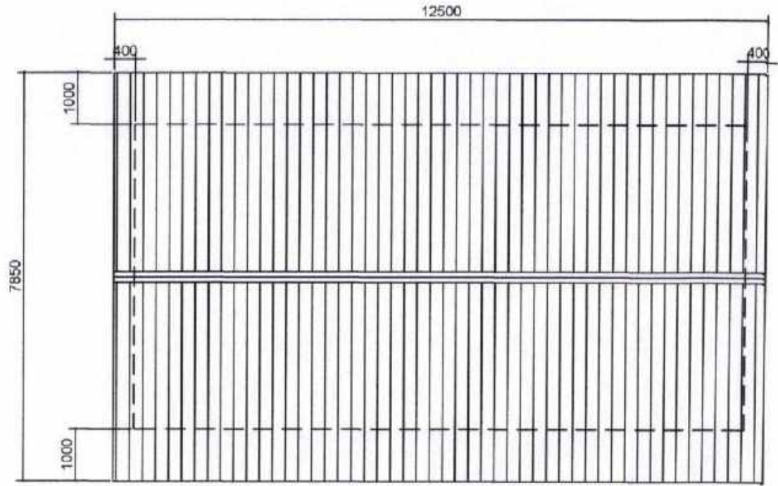
○ R O O F P L A N SCALE: N T S
