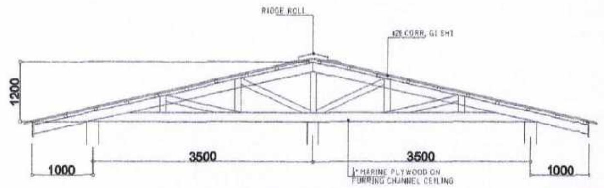
TRUSS DET. SCALE: 1/20PTS
