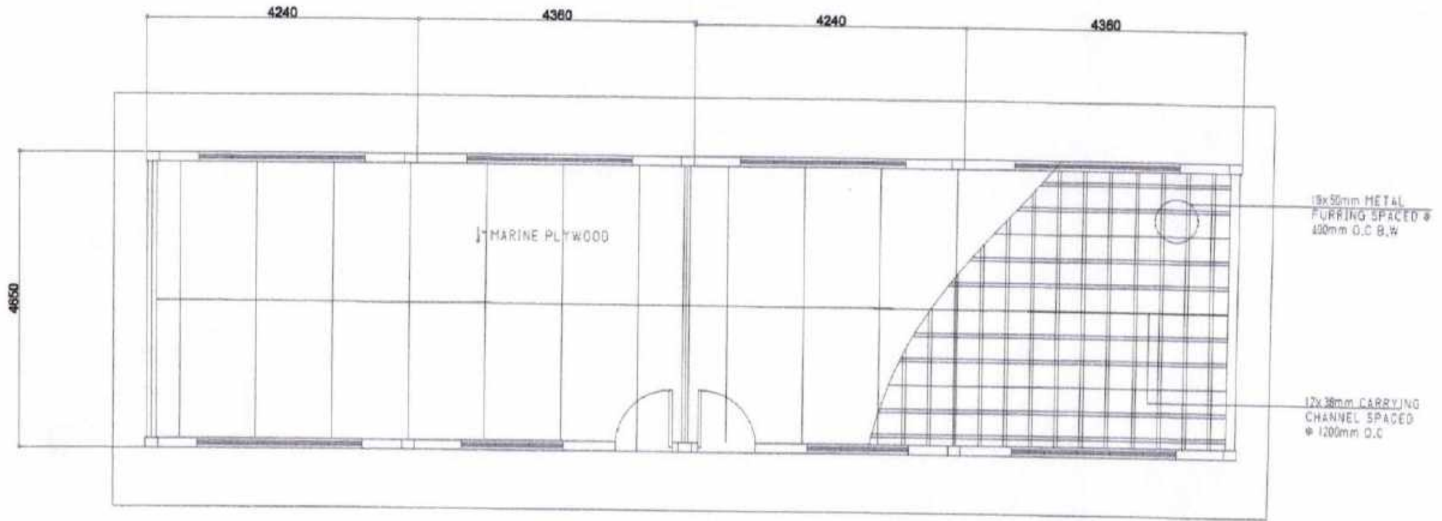
CEILING PLAN SCALE: 1/2011
