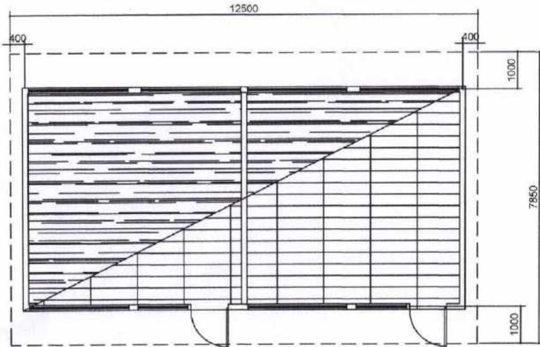
○ C E I L I N G P L A N SCALE: N T S
