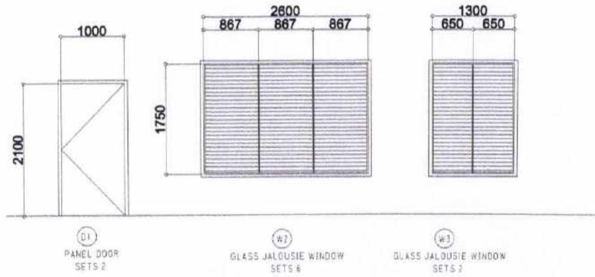
DOORS & WINDOWS SCHEDULE SCALE: 1:25M.T.S
