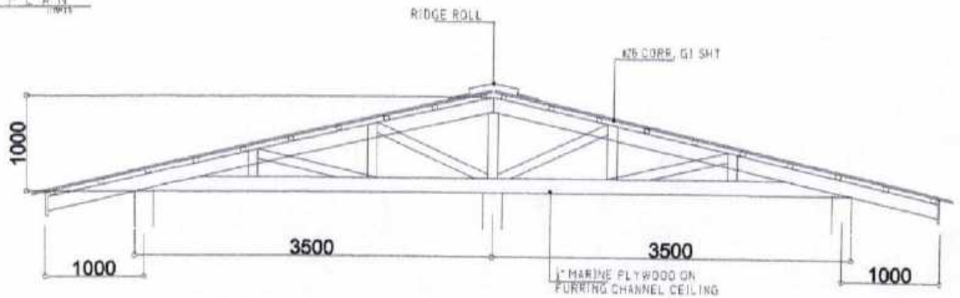
TRUSS DET. SCALE: 1:25 H.T.S.
