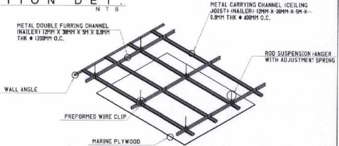
○ CEILING DET. SCALE: N T S
