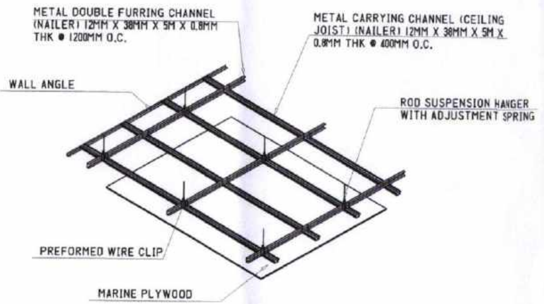
CEILING DET. SCALE: N T S
