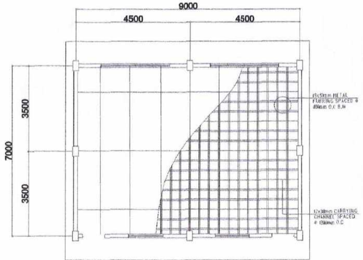
CEILING PLAN SCALE: 1:200
