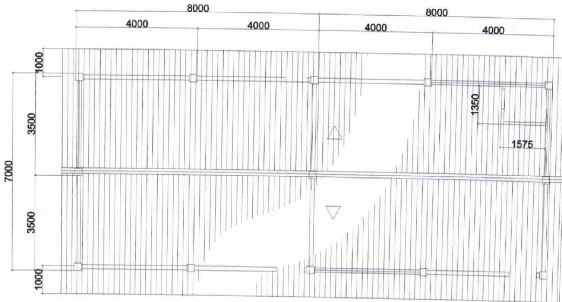
ROOF PLAN SCALE: 1:200
