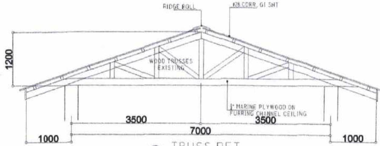
TRUSS DET. SCALE: 1:25MTS
