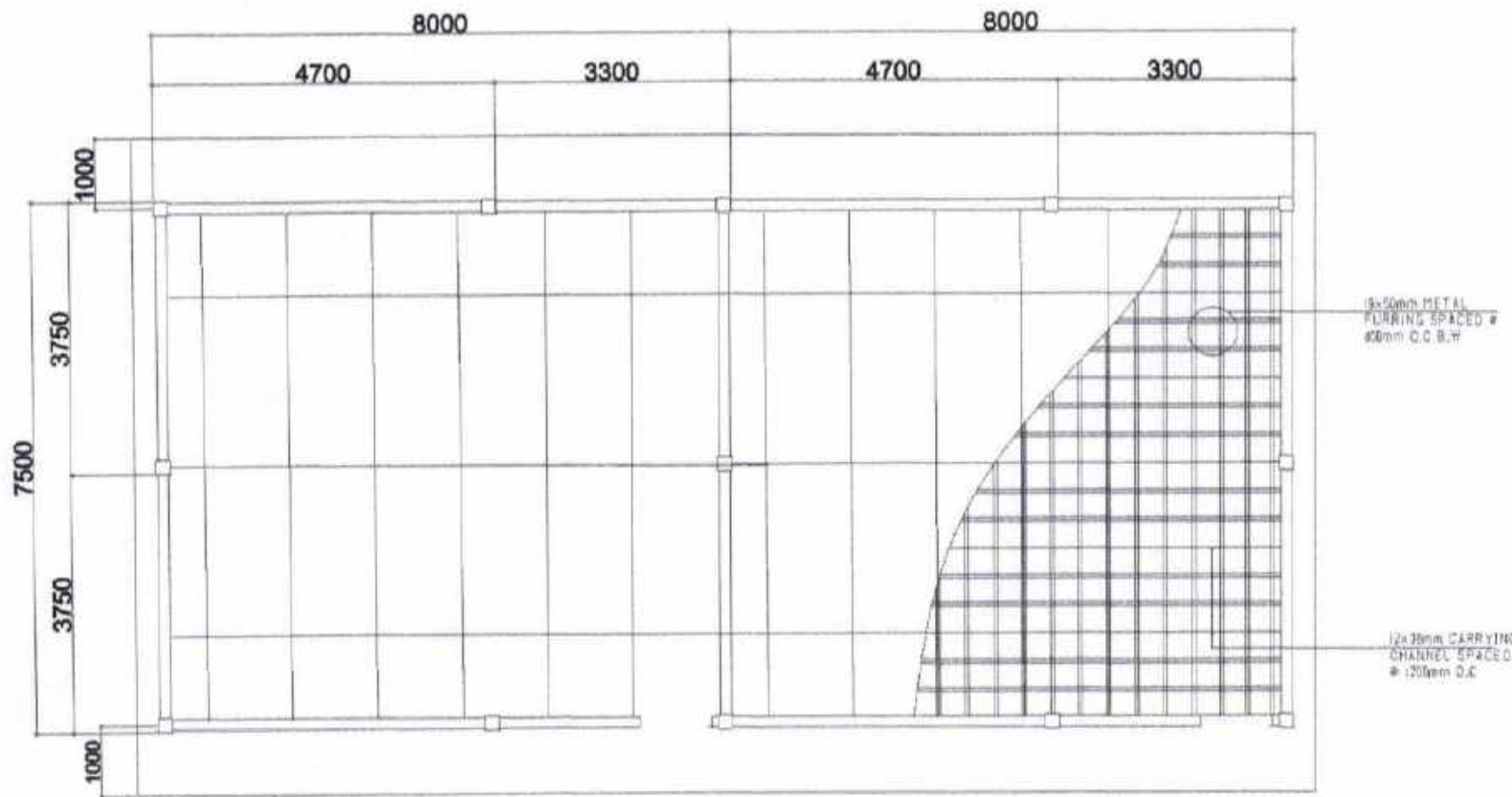
CEILING PLAN SCALE: 1:50
