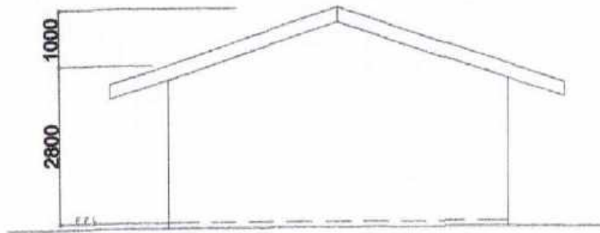
RIGHT SIDE ELEV. SCALE: 1/4"=1'-0"
