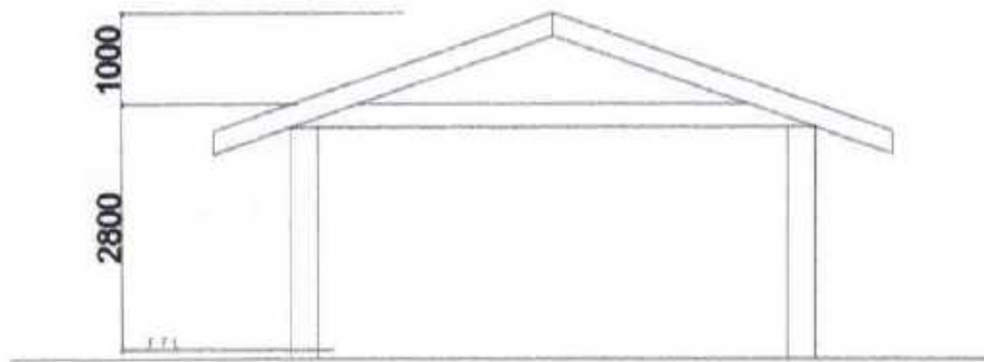
RIGHT SIDE ELEV. SCALE: 1/8"=1'-0"
