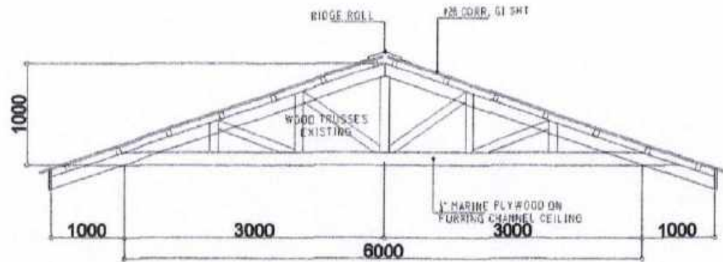
TRUSS DET. SCALE: 1/4"=1'-0"
