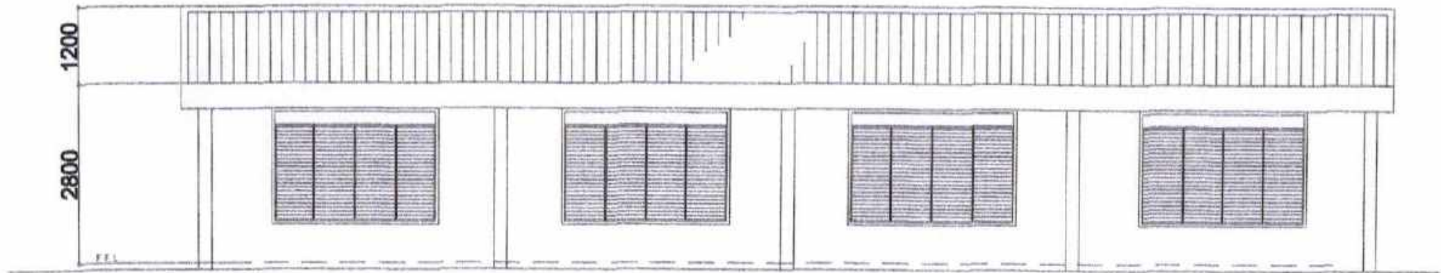
REAR ELEVATION SCALE: 1/8"=1'-0"
