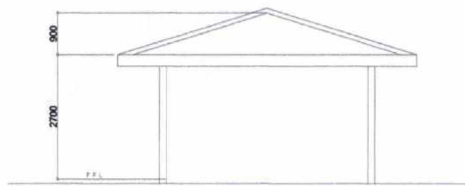
RIGHT SIDE ELEV. SCALE: 1/8"=1'-0"
