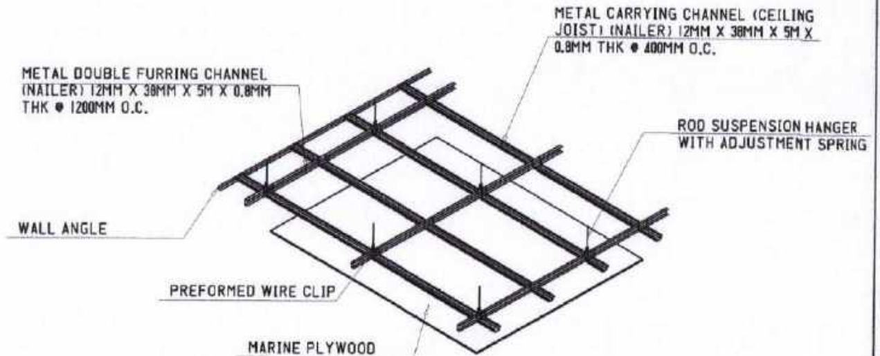
○ CEILING DET. SCALE: N T S
