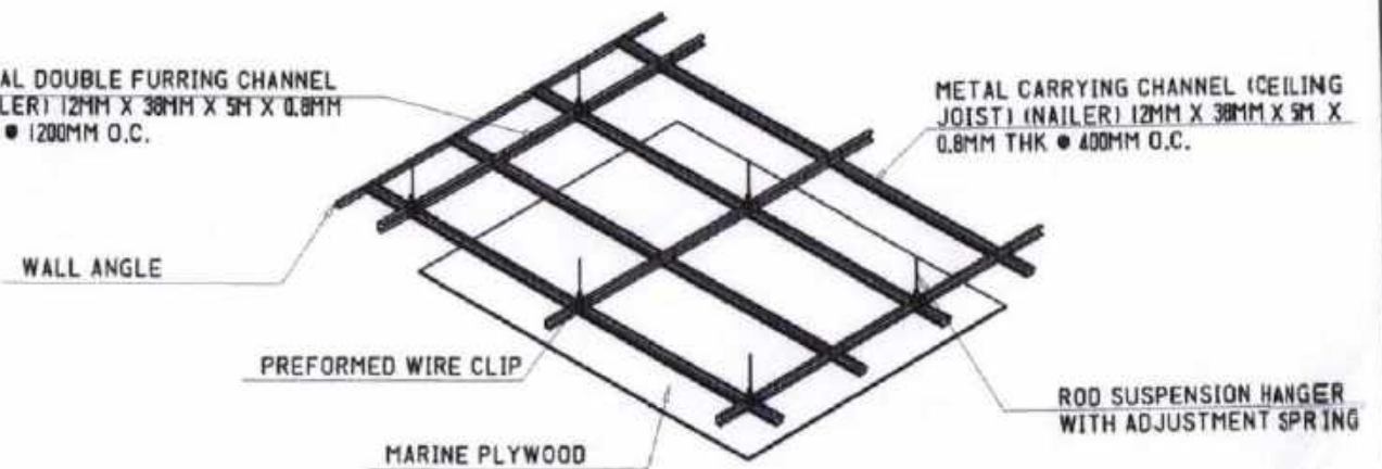
CEILING DET. SCALE: N T S
