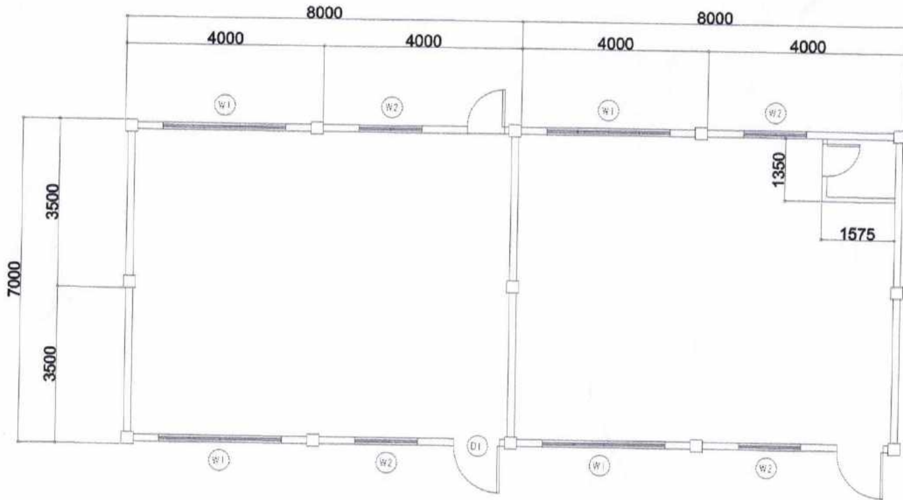
EXISTING FLOOR PLAN SCALE: 1:200
