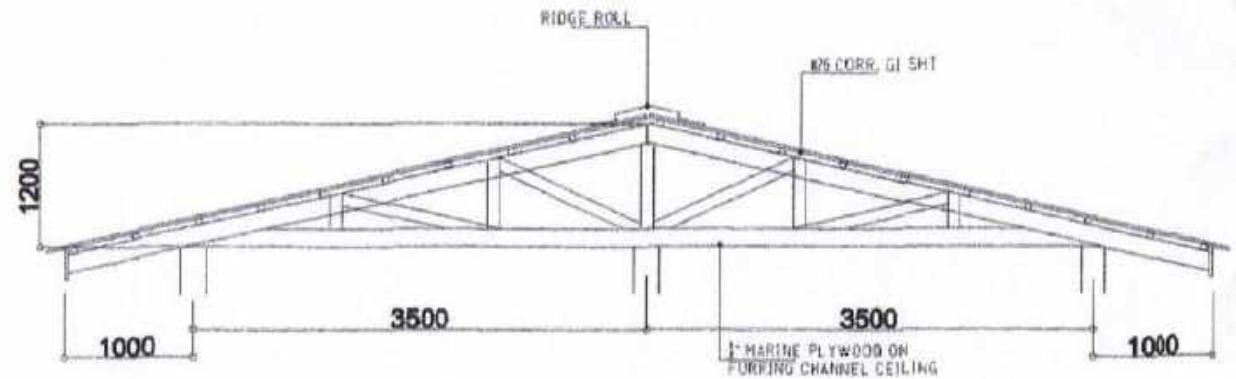
TRUSS DET. SCALE: 1/25HTS
