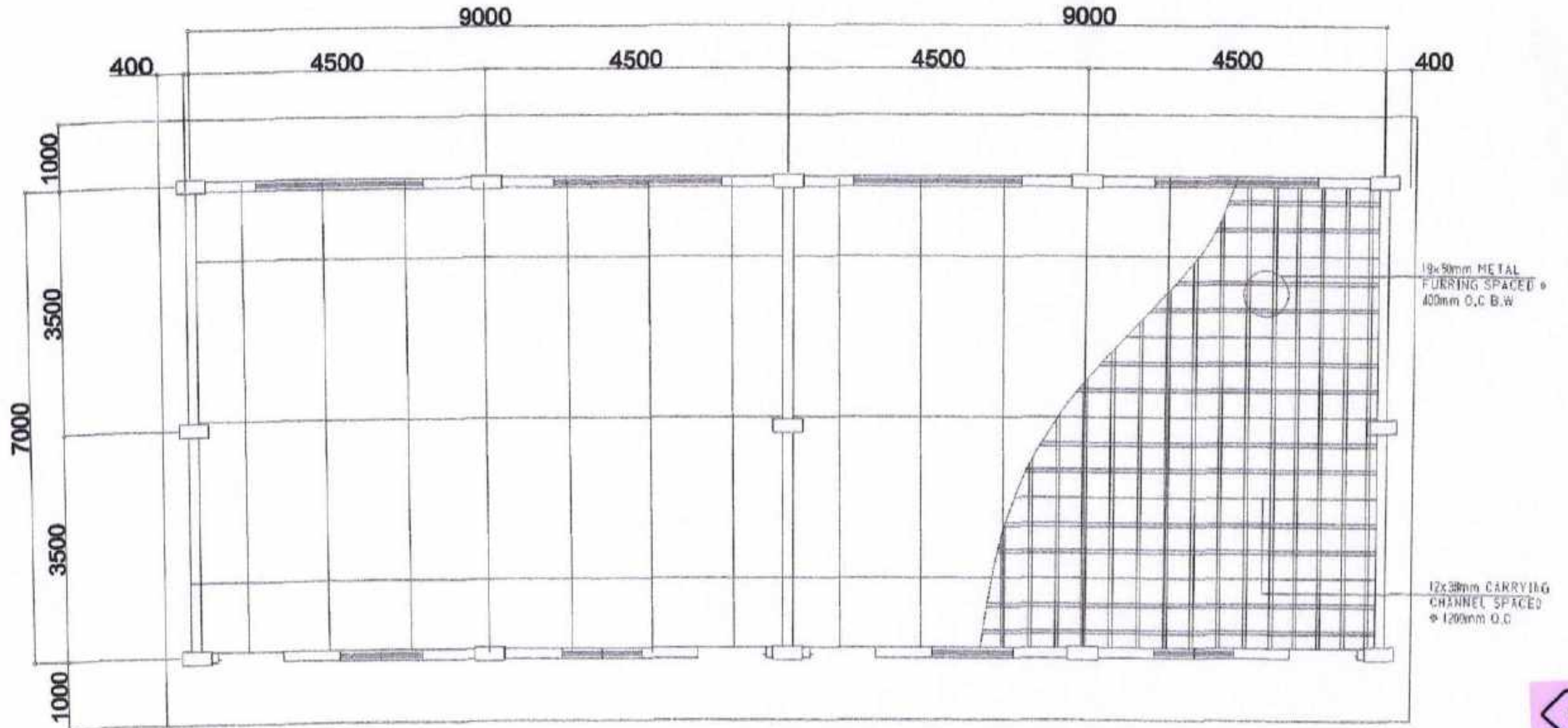
CEILING PLAN SCALE: 1/8"=1'-0"
